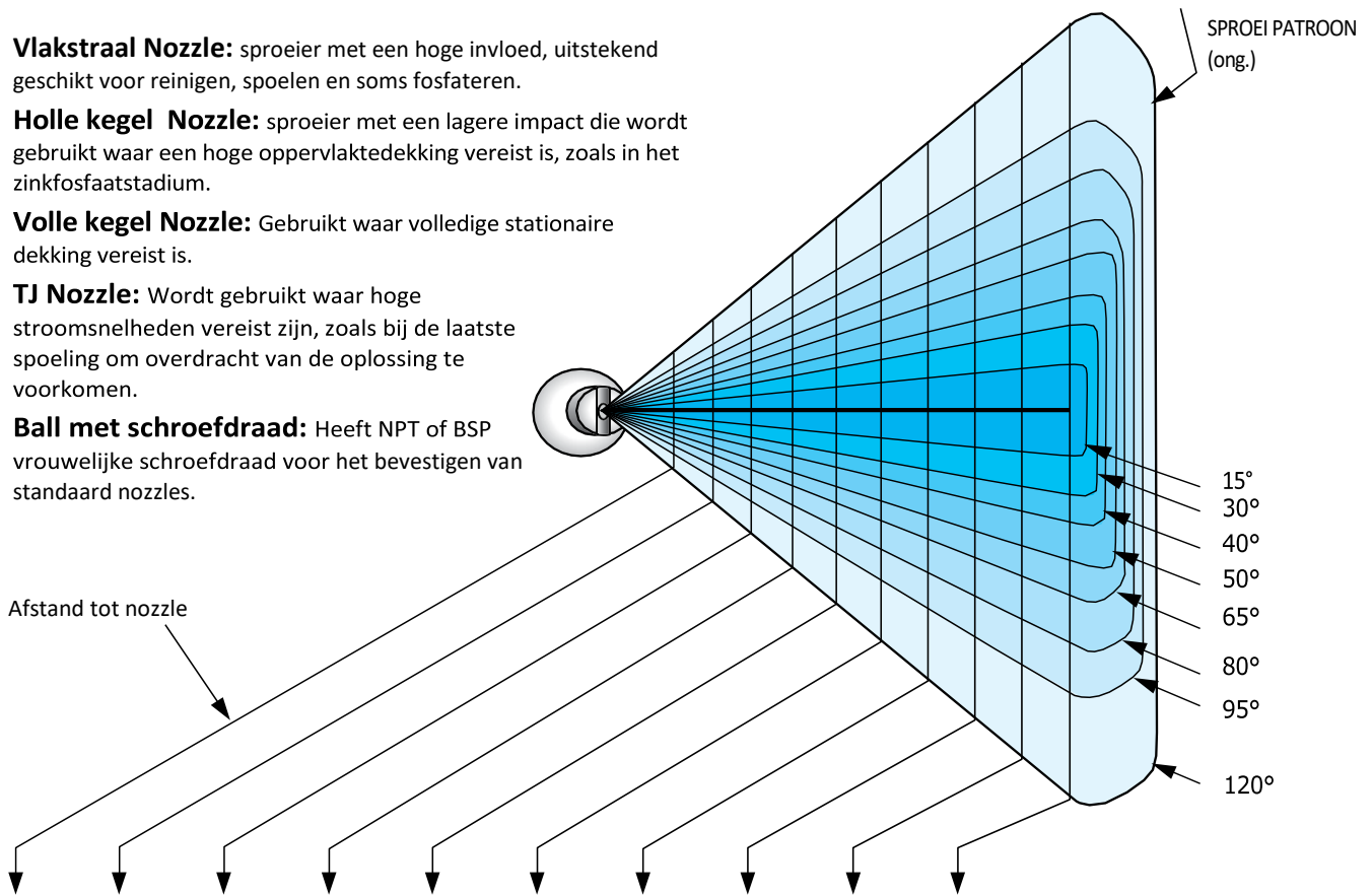
BREEDTE SPROEIPATROON (CM) AFHANKELIJK VAN DE HOOGTE
